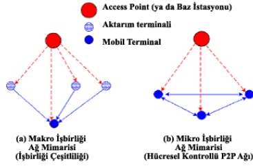
Şekil 6. İşbirlikçi Ağ Mimarîleri
