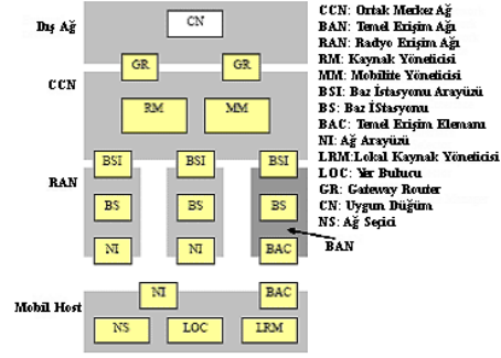
Şekil 3. Heterojen Wireless Ağ Mimarîsi
