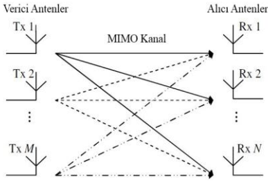
Şekil 3. MIMO kanal yapısı
