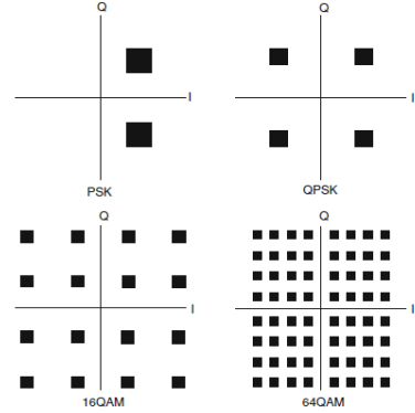
Şekil 5. Dijital modülasyon teknikleri
