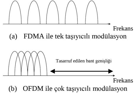
Şekil 7. FDMA ve OFDM karşılaştırması
