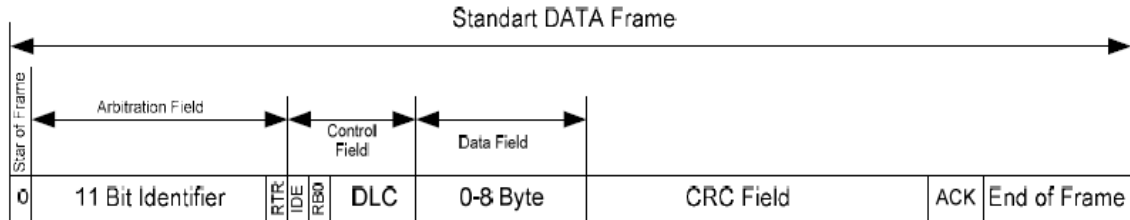
Şekil 1. Kontrol Alan Ağı Standart Data Frame
