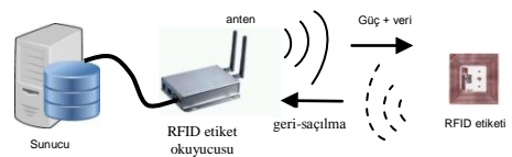
Şekil 2. Pasif UHF RFID Sistemi
